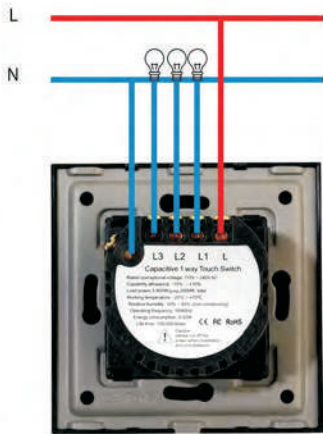
1way/Bell wiring
