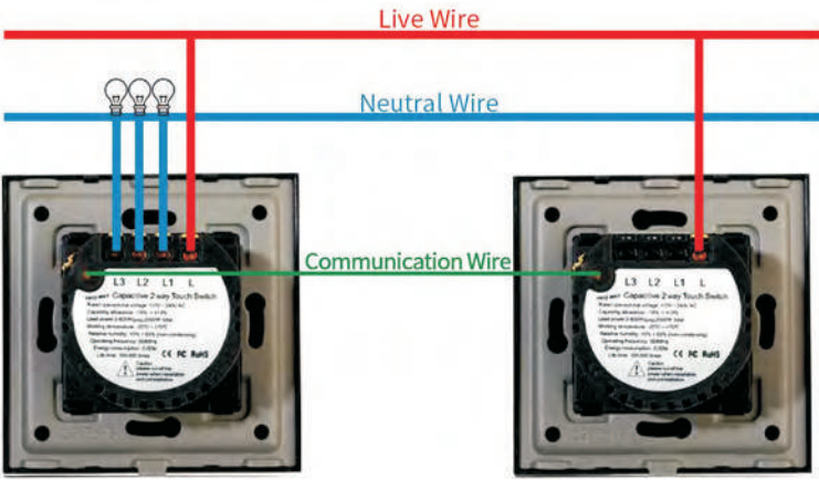
2way wiring
